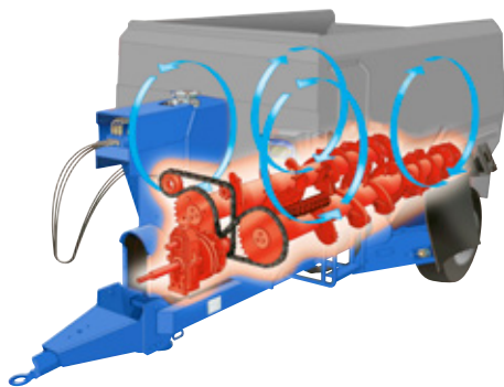
System rozdrabniająco-mieszający DUO MIX
